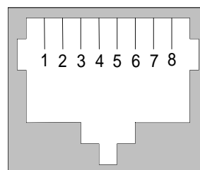
RJ45
