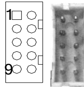
USB3/USB4
