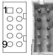
USB5/USB6
